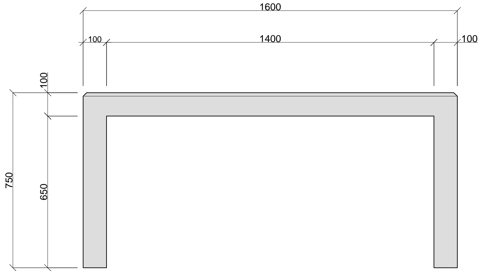
ELEVATION
