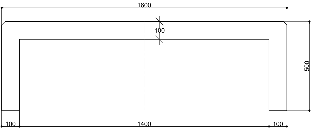
ELEVATION
